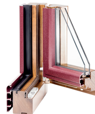
profilo legno/alluminio Soft Line della serie UNIFORM
