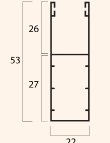
Guida in alluminio estruso A53 22 x 53 mm
