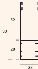
Guida in alluminio estruso A80 28 x 80 mm
