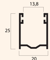
Guida in alluminio estruso A25 20 x 25 mm
