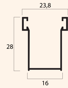
Guida in alluminio estruso A16 16 x 28 mm
