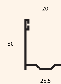
Guida in alluminio estruso A27 25,5 x 30 mm
