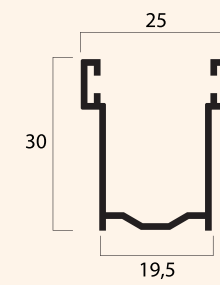
Guida in alluminio estruso A30 19,5 x 30 mm
