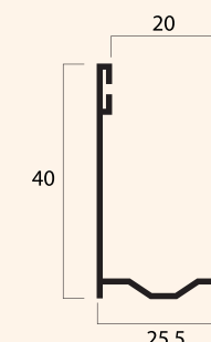
Guida in alluminio estruso A40 25,5 x 40 mm
