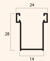
Guida in alluminio estruso A14 14 x 28 mm
