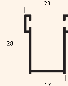
Guida in alluminio estruso A28 17 x 28 mm
