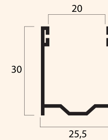
Guida in alluminio estruso A27 25,5 x 30 mm
