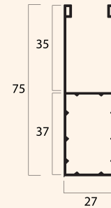
Guida in alluminio estruso A75 27 x 75 mm
