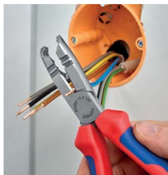
Taglia quando si accorciano conduttori singoli
