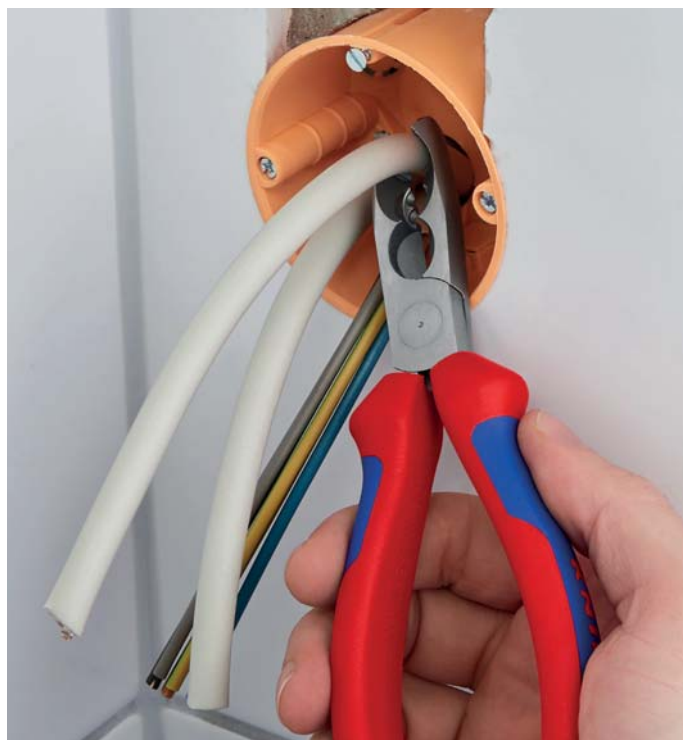
Spelatura guaina anche in profondità nella cassetta di derivazione a incasso
