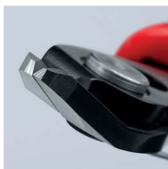
Sezione di taglio con micro-spostamento dei taglienti controllato per un taglio ultrapreciso anche dei fili metallici più sottili e per una lunga durata
